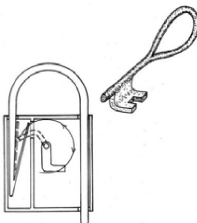
Hänglås med spärrfjädrar och vridnyckel från vikingatid
